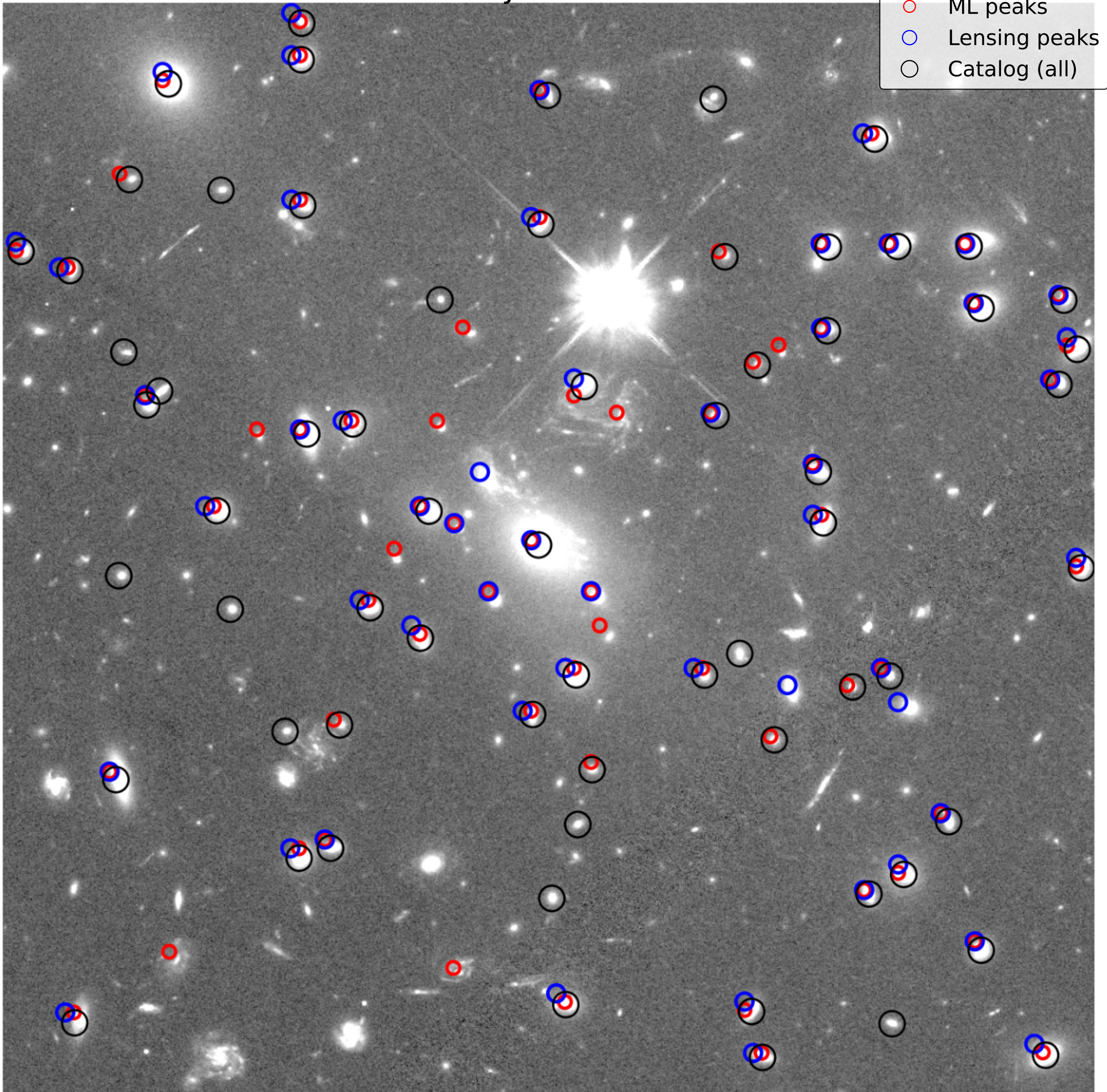
MACS J1149+2223
